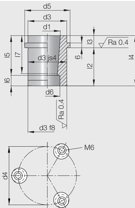
I7: Säule Konus/Pillar taper I7= I5 - 1mm
